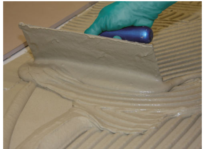
Geschmeidiges Aufziehen des Kammбетtes des fließfähigen Sopro FKM XL.
